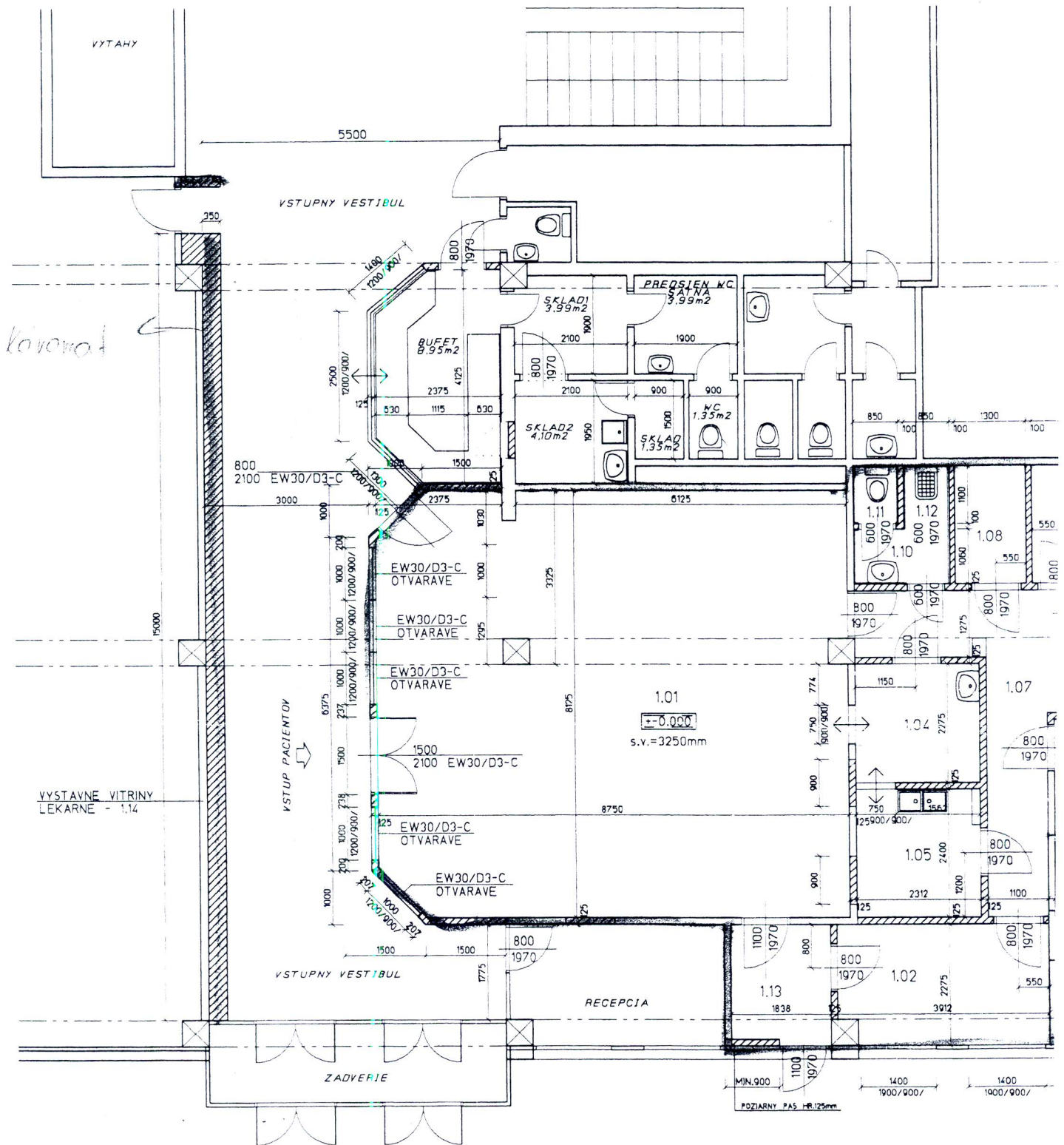
PODORYS M=1:100
