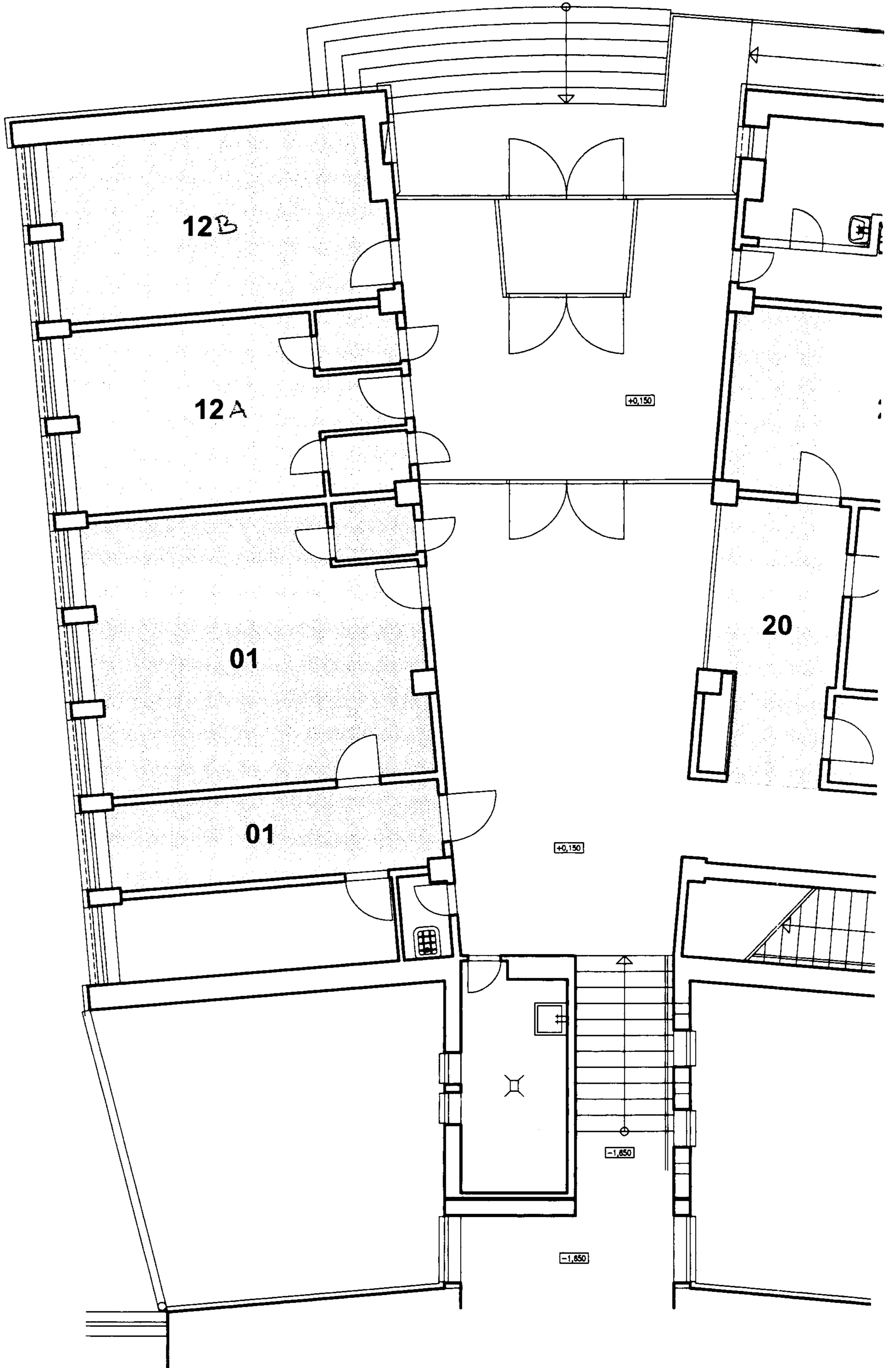
PAVILÓN "D" - PÔDORYS PRÍZEMIA M=1:100
