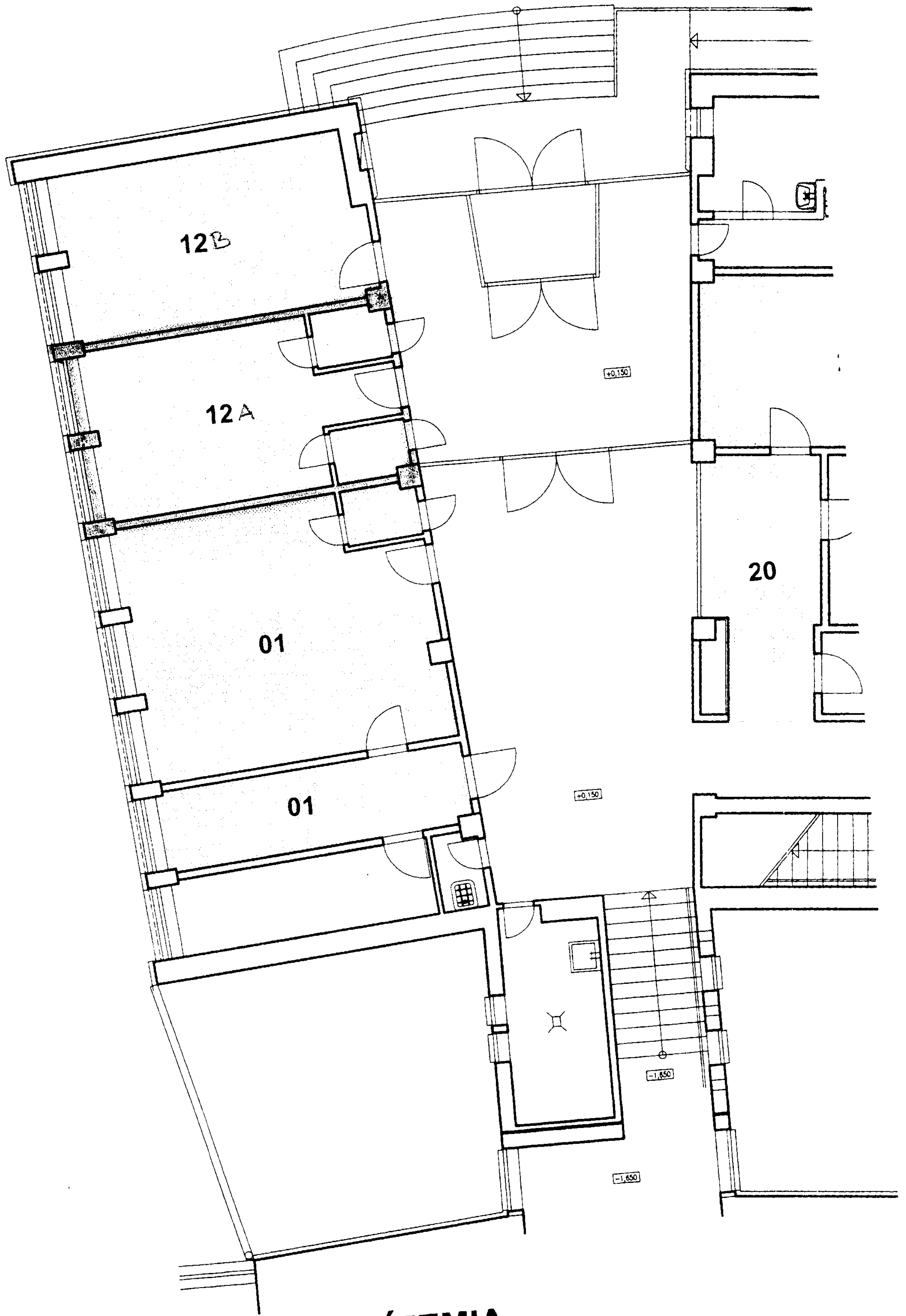
PAVILÓN "D" - PÔDORYS PRÍZEMIA M=1:100
