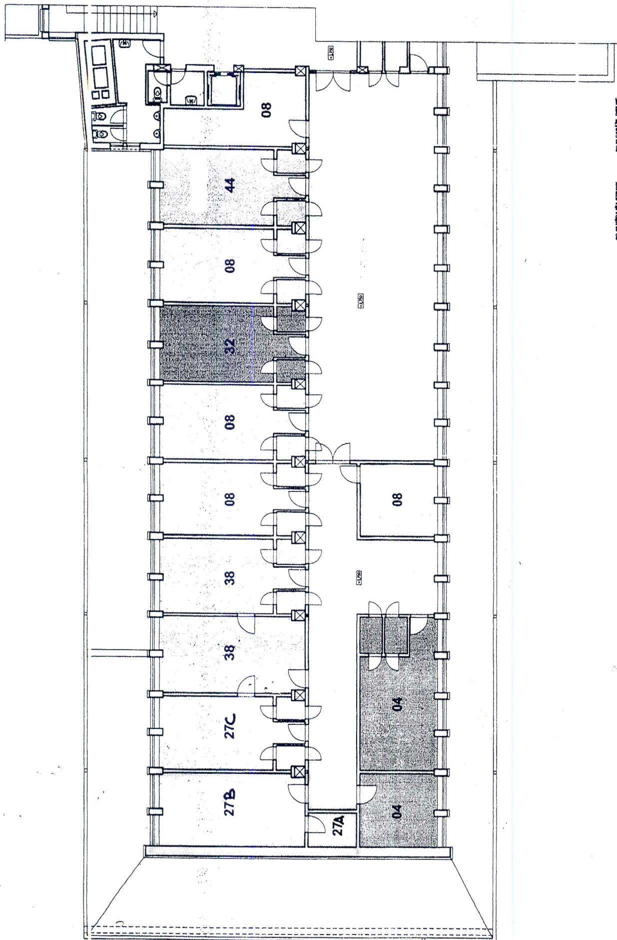
PAVILÓN "A" - PÓDORYS 1.POSCHODIA M=1:120
